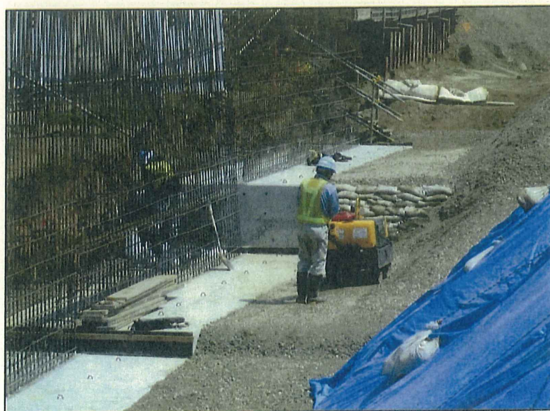
埋戻し (底板コンクリート打設後)
